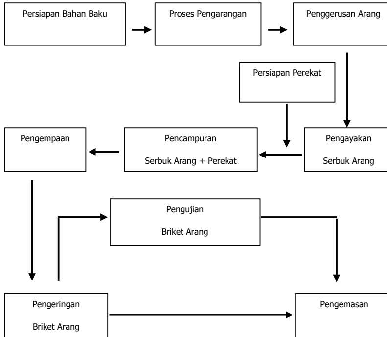
Gambar 1. Tahapan Proses Pembuatan Briket Arang
